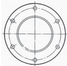
FLANGE / FLANGES / BRIDES / FLANSCHEN
